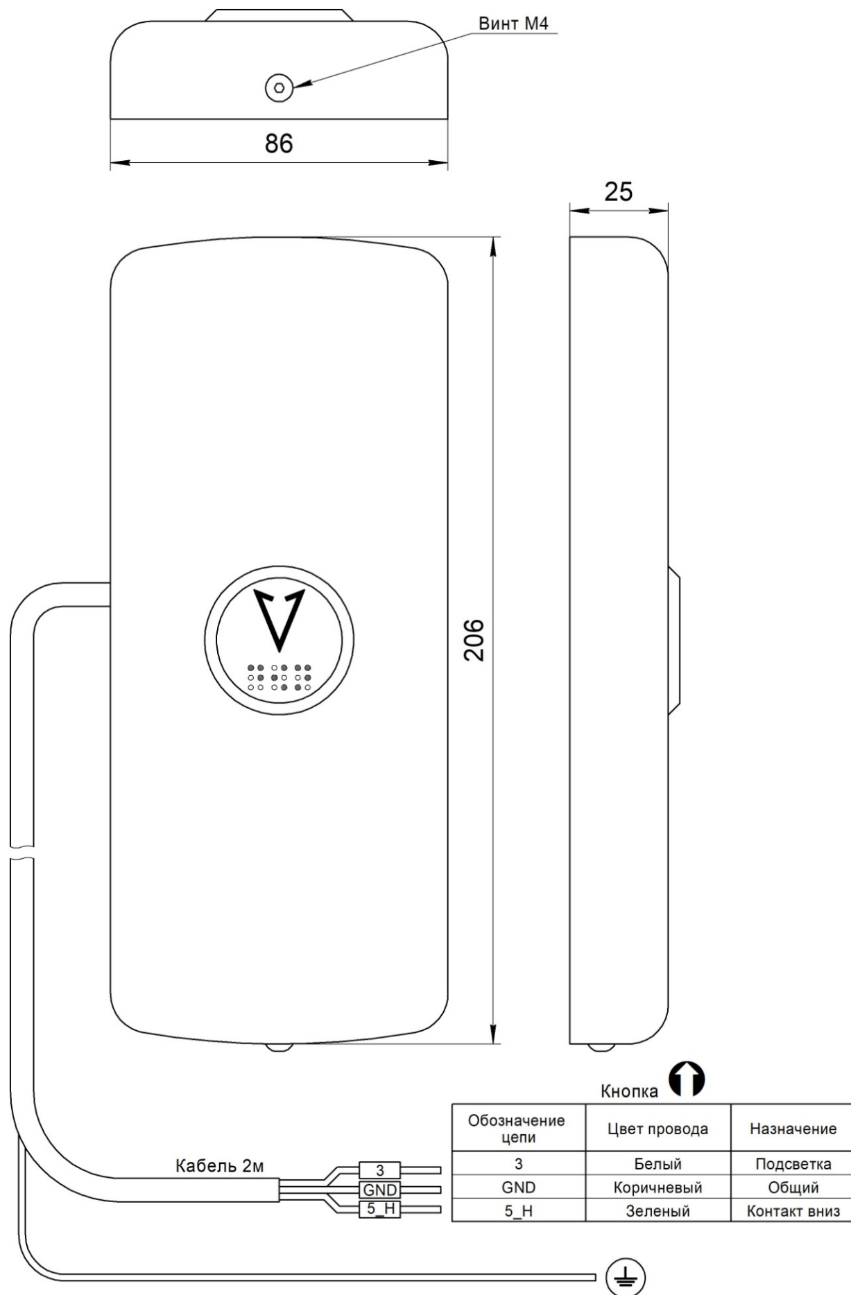
Рис.1 Внешний вид и габаритные размеры Вызывного поста ВП-1102-03
